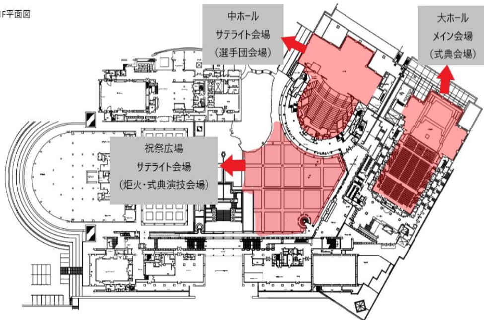
B1平面図
